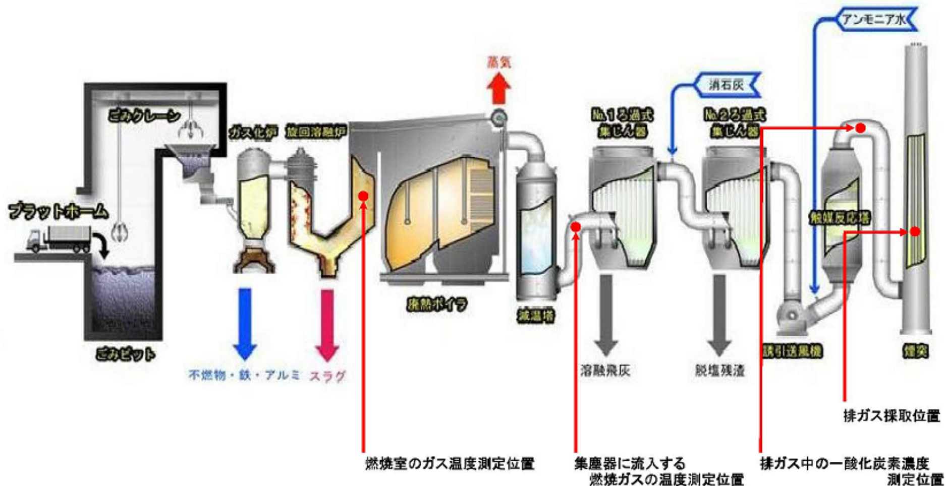
各種測定位置及び排ガス採取位置図
